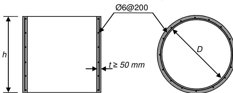
គំនូសបង្ហាញបច្ចេកទេសកង់លូអណ្ណាច
