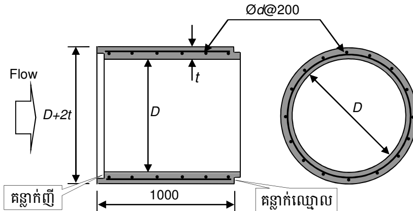
គំនូសប្លង់បច្ចេកទេសកង់លូមូលដោះទឹក
