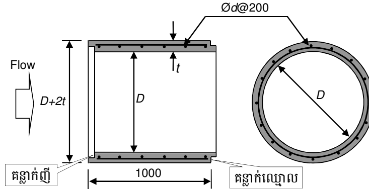
គំនូសប្លង់បច្ចេកទេសកង់លូមូល
